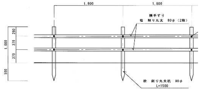
防護柵構造図
