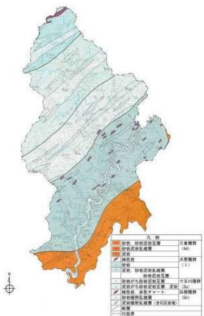
【地質図】
