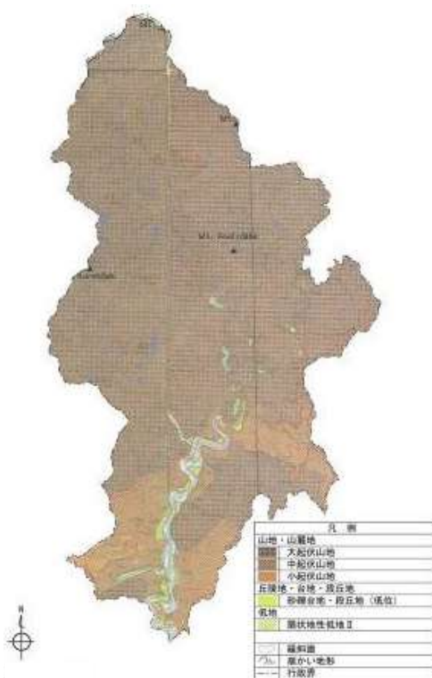
【地形区分図】
