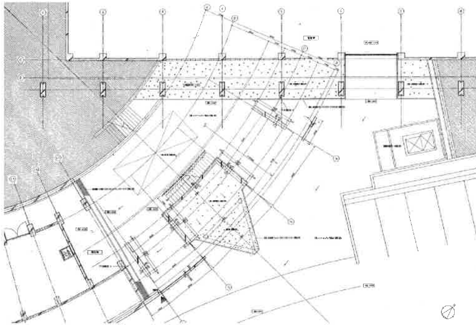
< 1 階 >
